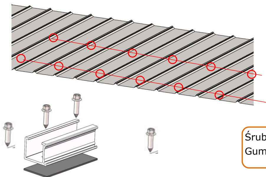
Mini-szyna pozioma
